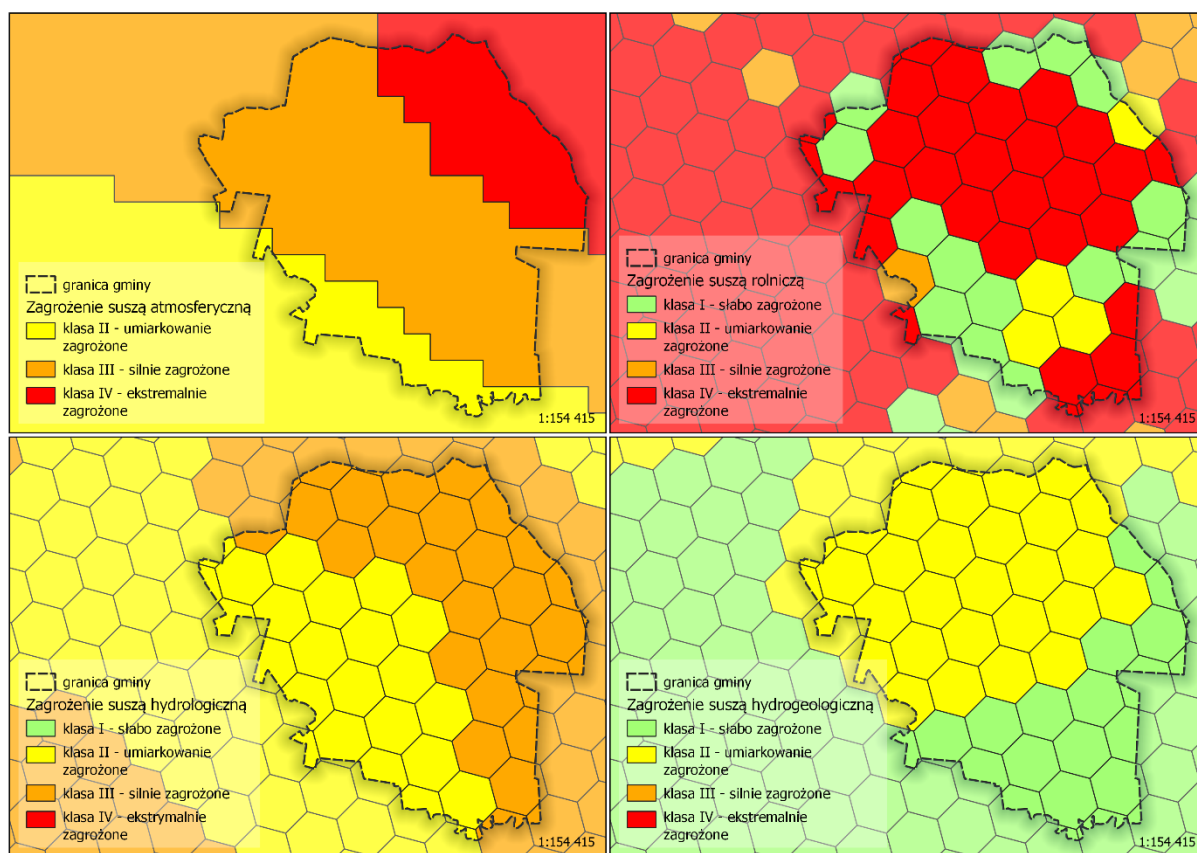
Rysunek 4. Stopień zagrożenia suszą według jej typów: atmosferyczna, rolnicza, hydrologiczna oraz hydrogeologiczna
